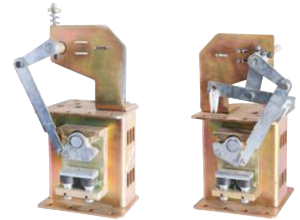
Ловители плавного торможения 9 мм/ 16 мм Progressive Safety Gear 9 mm / 16 mm
